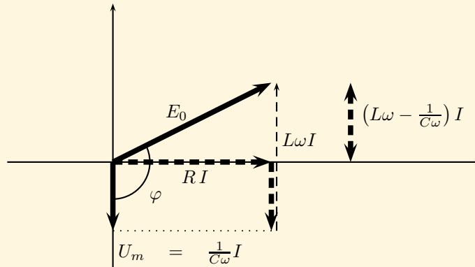
Diagramme de Fresnel
