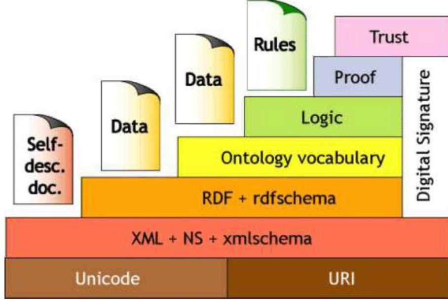
الشكل (1) يبين طبقات شبكة الويب الدلالية
