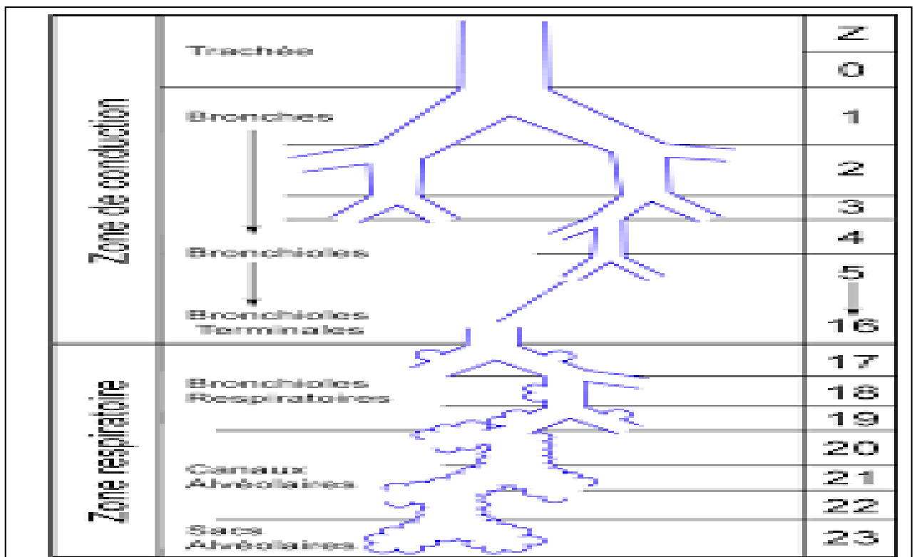
Fig.4 : Schéma de la division dichotomique de l’arbre trachéo-bronchique.
