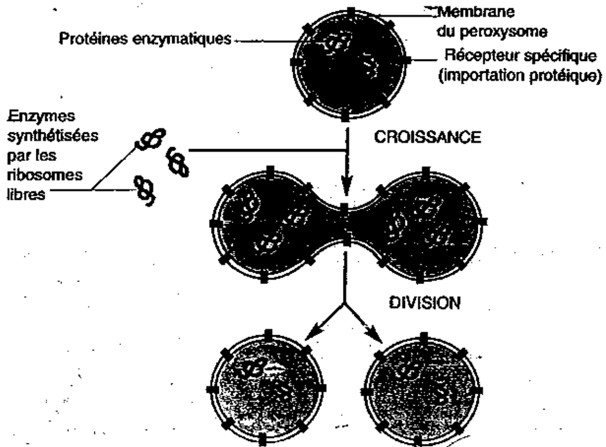
Figure 5 : Biogenèse des peroxysomes
