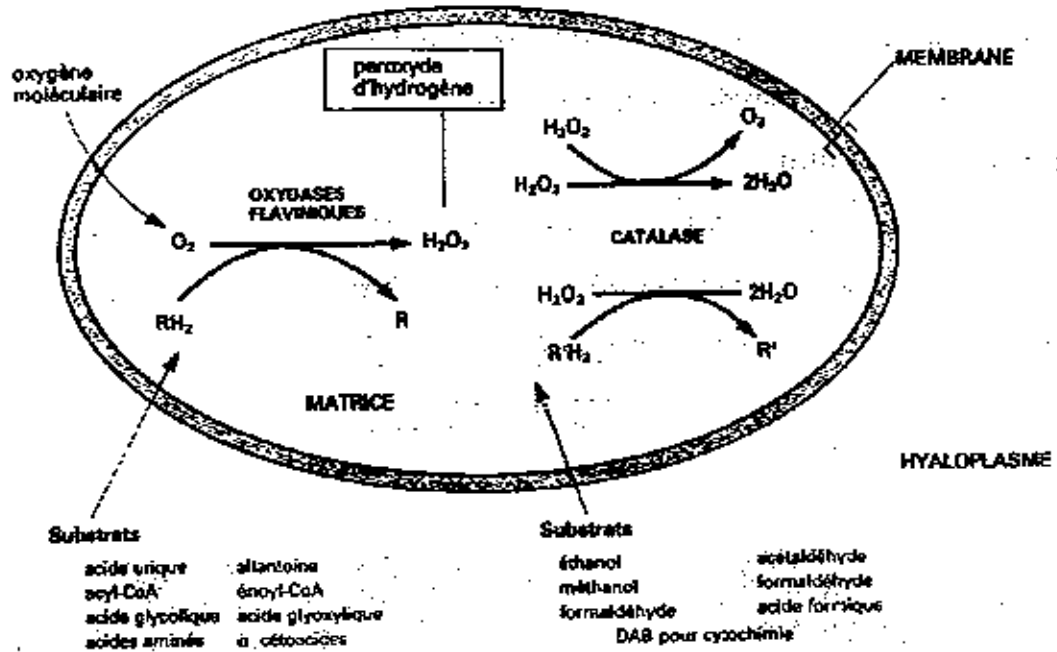
Figure 3 : Réaction d'oxydation et de peroxydation dans les peroxysomes
