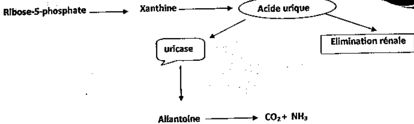
Figure 4 : Métabolisme simplifié de l'acide urique
